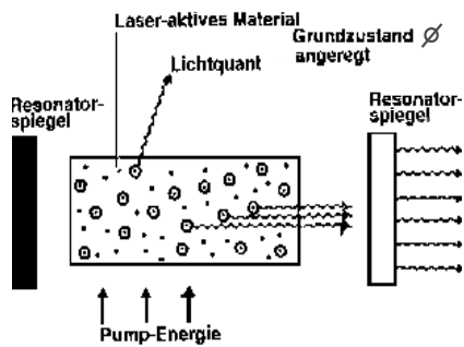
Aufbau eines Lasers (schematisch)
