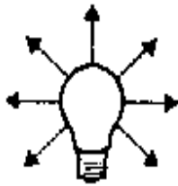
Divergenz bei gewöhnlichem Licht
